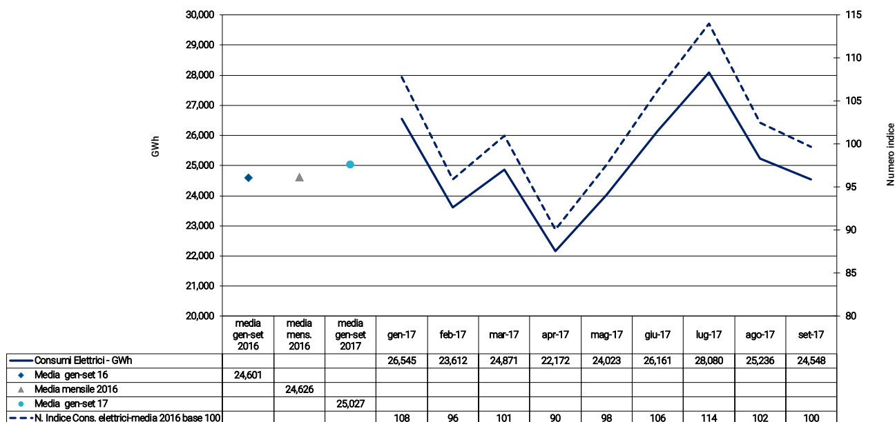
Consumi elettrici
