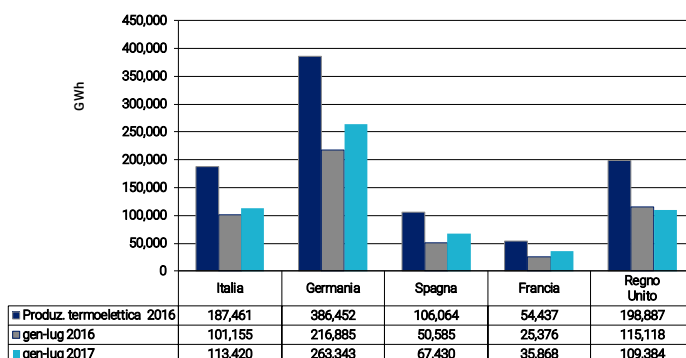
Produzione termoelettrica
