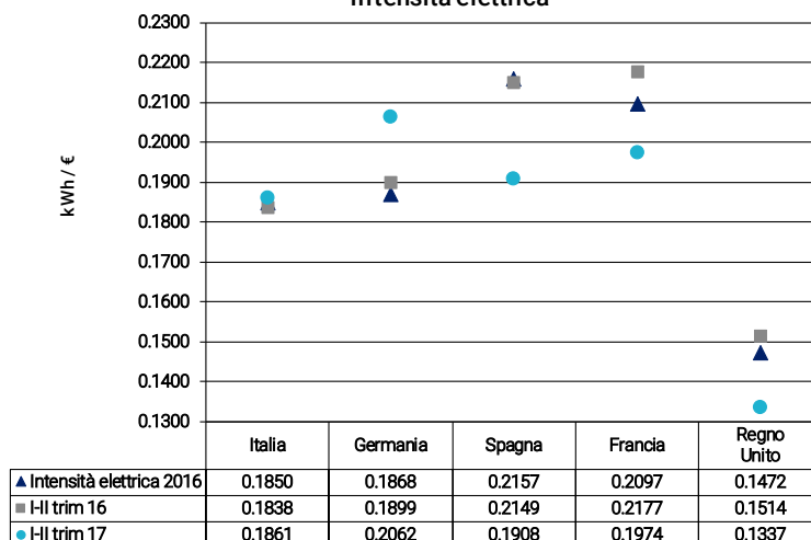
Intensità elettrica
